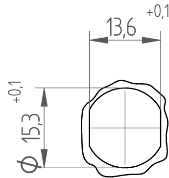
Montageöffnung Installation opening
